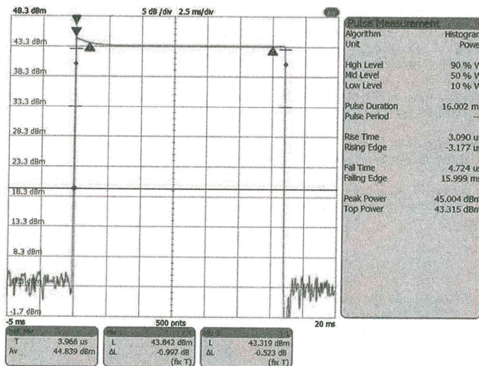
Рис.5. Эпюра радиоимпульса на выходе передающего канала МППУ
